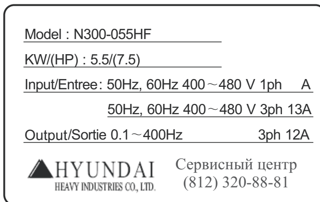
Рисунок 1-2 Содержание фирменной таблички
